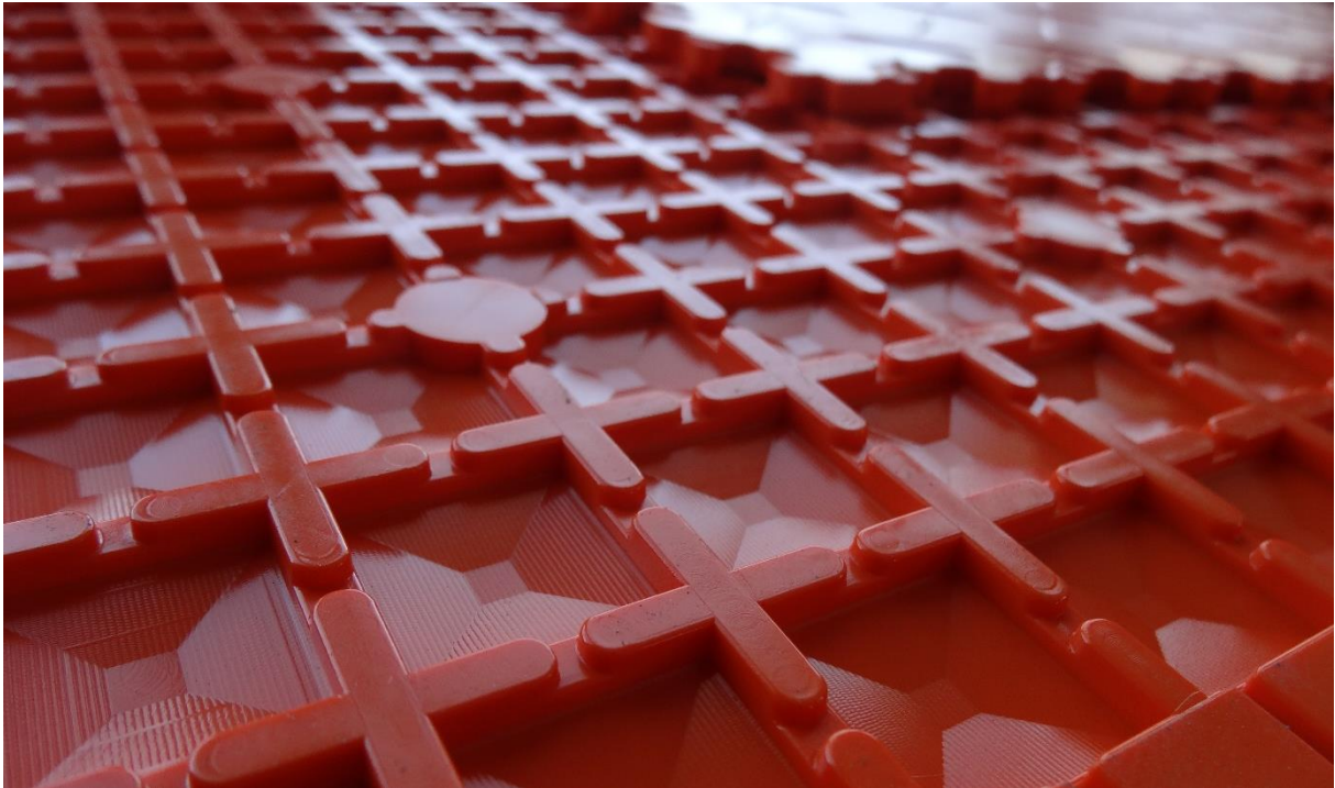
Die untere Seite der Fliese Fortelock Light nach der Entwicklungsmodifizierung. Pyramidensystem.
